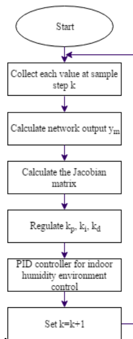
3.1-сурет- RBFNN-ПИД-реттегіштің технологиялық схемасы
