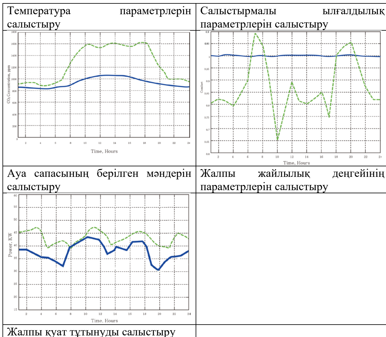
Сурет 4.1-Эксперимент нәтижелері. Жасыл сызық: дәстүрлі жүйе; көк сызық: ұсынылған жүйе
