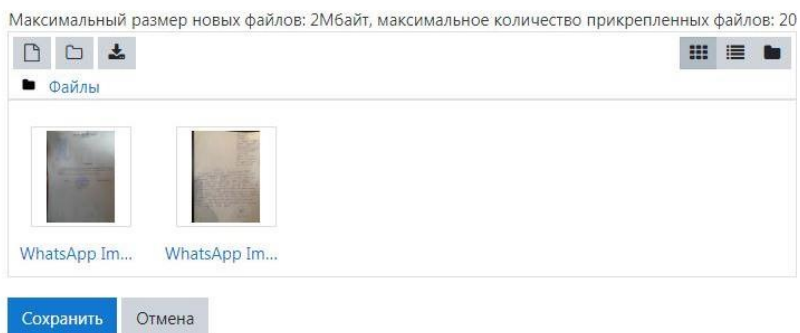
Рисунок 8. Добавление файлов.
