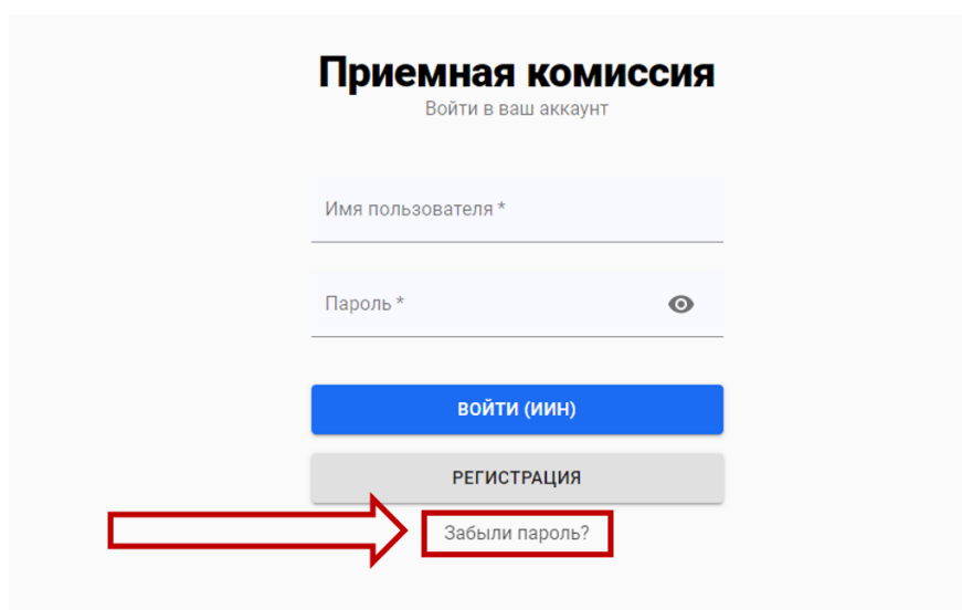
Рисунок 9. Сброс пароля
